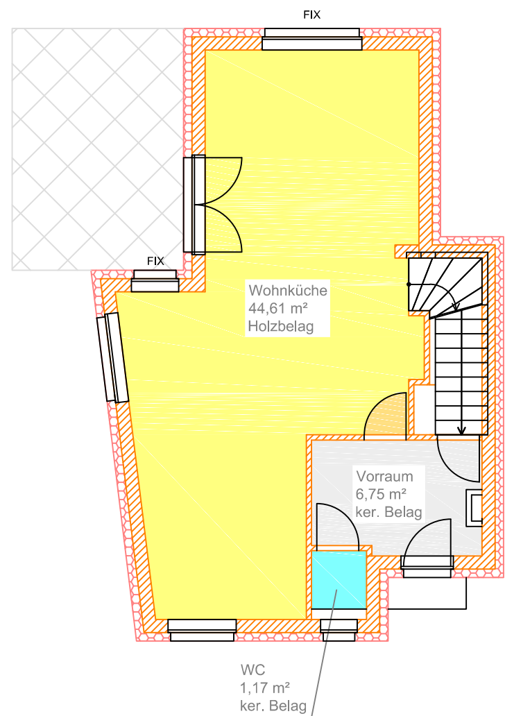
Erdgeschoß 1:100
